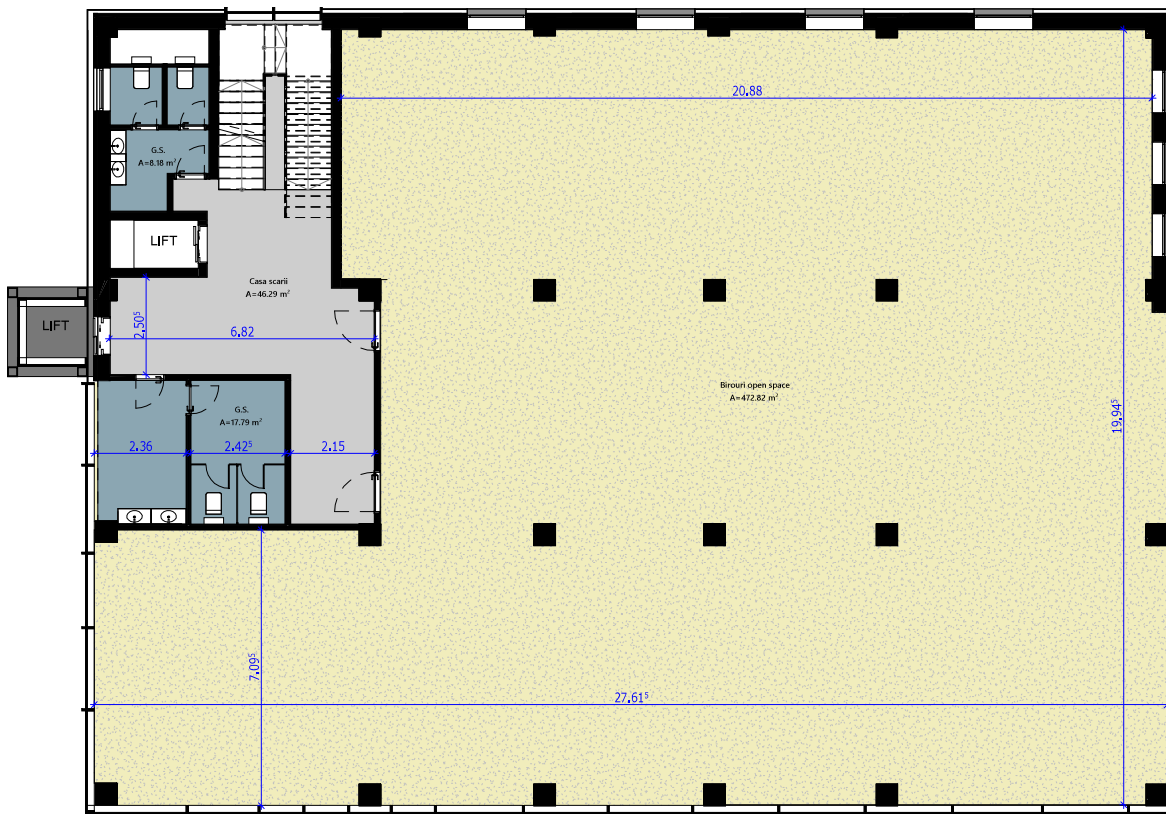
PLAN ETAJ 8 SCARA: 1 : 100
