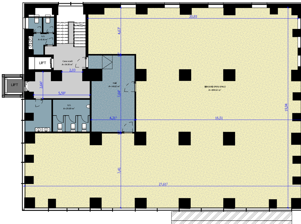
PLAN ETAJ 5 SCARA: 1 : 100
