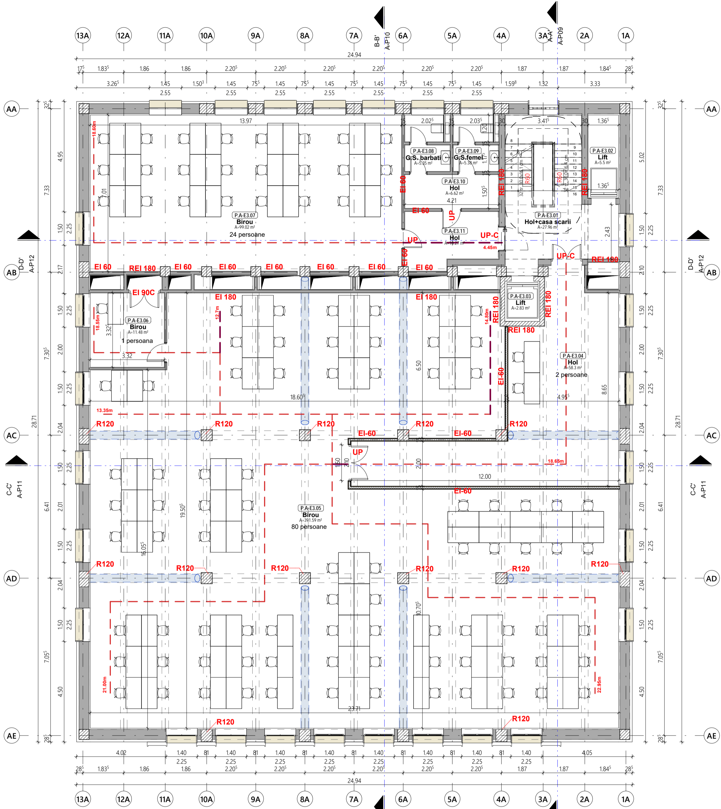
6 ETAJ III CORP A PROPUS SCARA: 1 : 100
