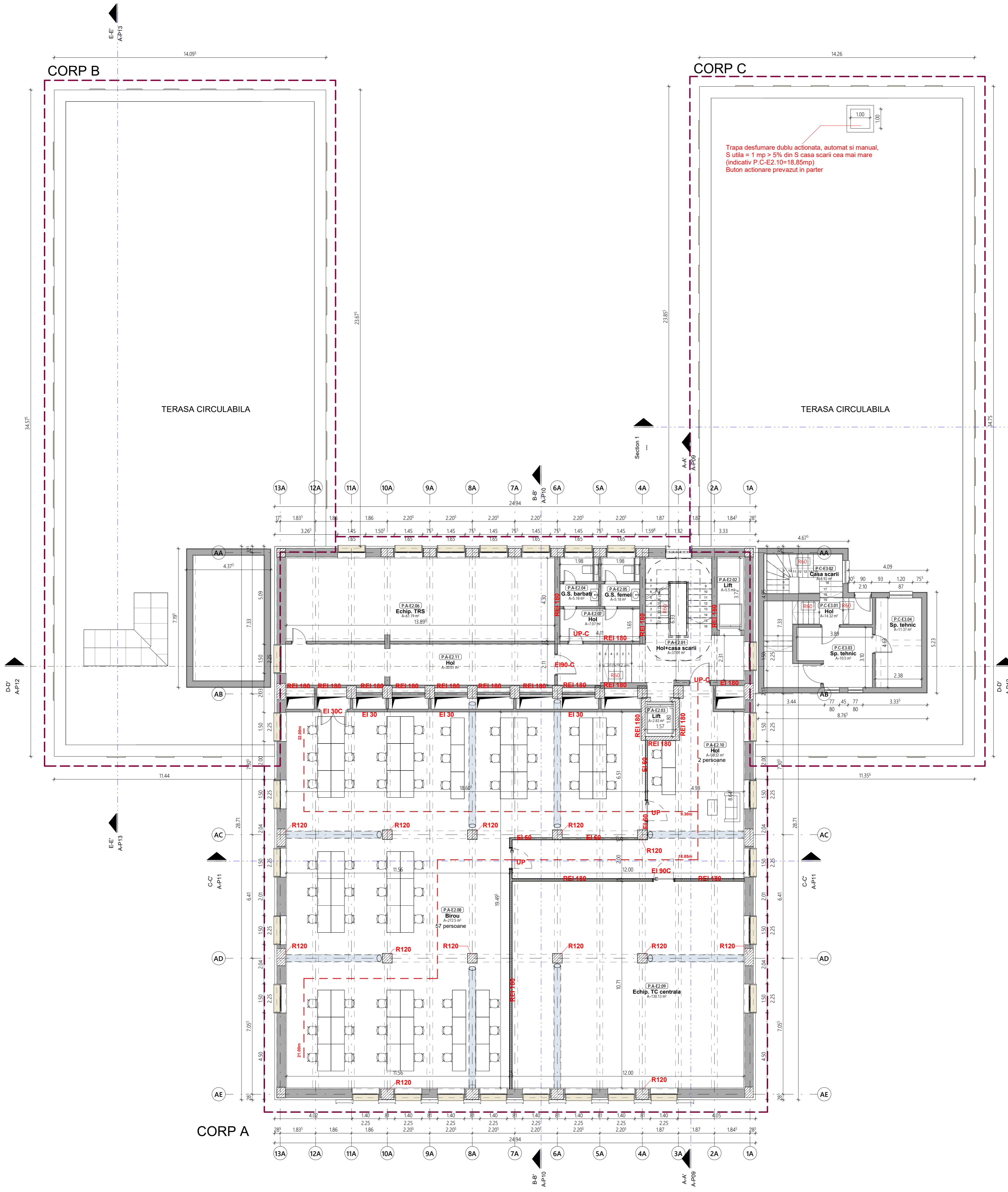
5 ETAJ II CORP A PROPUS SCARA: 1 : 100
